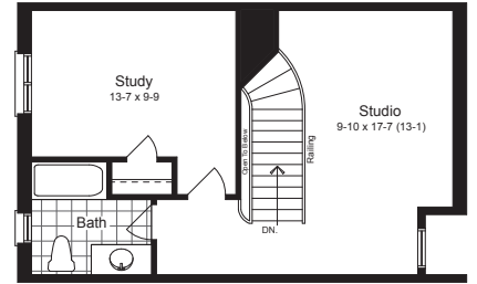
Optional Loft
